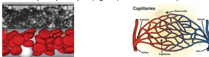
Figure 1 : Gauche – (a) expérience en quasi-2D et (b) simulation d'une suspension de GRs souples (rouge) et de GBs (blanc). Ceux-ci se localisent à la paroi. Droite – schéma typique d'un réseau vasculaire. Le sang s'écoule des artères vers les veines. A noter que les échanges avec l'environnement varient fortement entre les deux parties, rouge versus bleu.
