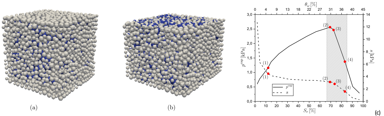
Figure 1: État initial (a) et final (b) d'un échantillon lors d'un essai triaxial. c) Contrainte capillaire moyenne Pcap [kPa] et succion s [kPa] en fonction du degré de saturation S_r [%] et de la teneur en eau volumétrique q_w [%] en bas et en haut de l'axe des x, respectivement.
