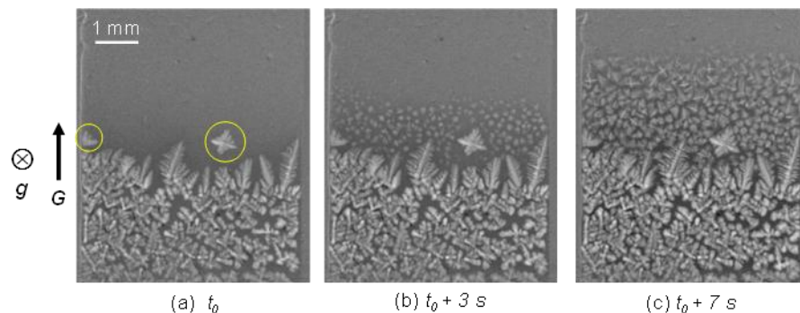
Figure 2 : Séquence de radiographies montrant la transition colonnaire équiaxe induite par un changement de la vitesse de refroidissement de R_1 = -0.032 \text{ °C/s} à R_2 = -2 \text{ °C/s} dans un alliage Al-10%pdsCu affiné et pour un gradient de température G = 3 \text{ °C/mm} .
